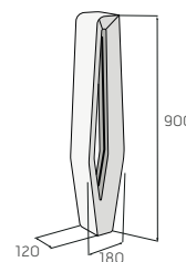
H-E-X – betonový sloupek s osvětlením
