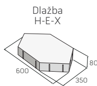
Vegetační dlažba H-E-X 80
