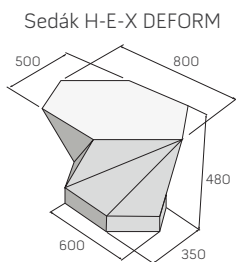
Sedák H-E-X DEFORM
