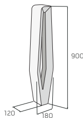
H-E-X – betonový sloupek
