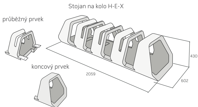
Stojan na kolo H-E-X
