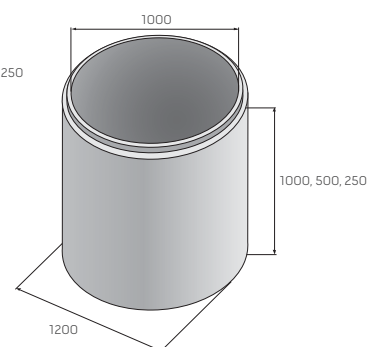
Betonová skruž TBX 2-100
