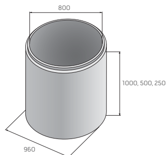
Betonová skruž TBX 2-80
