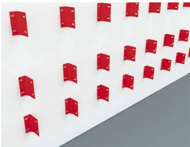
Obr. č. 2 Rozměření a rozmístění kotevních prvků
