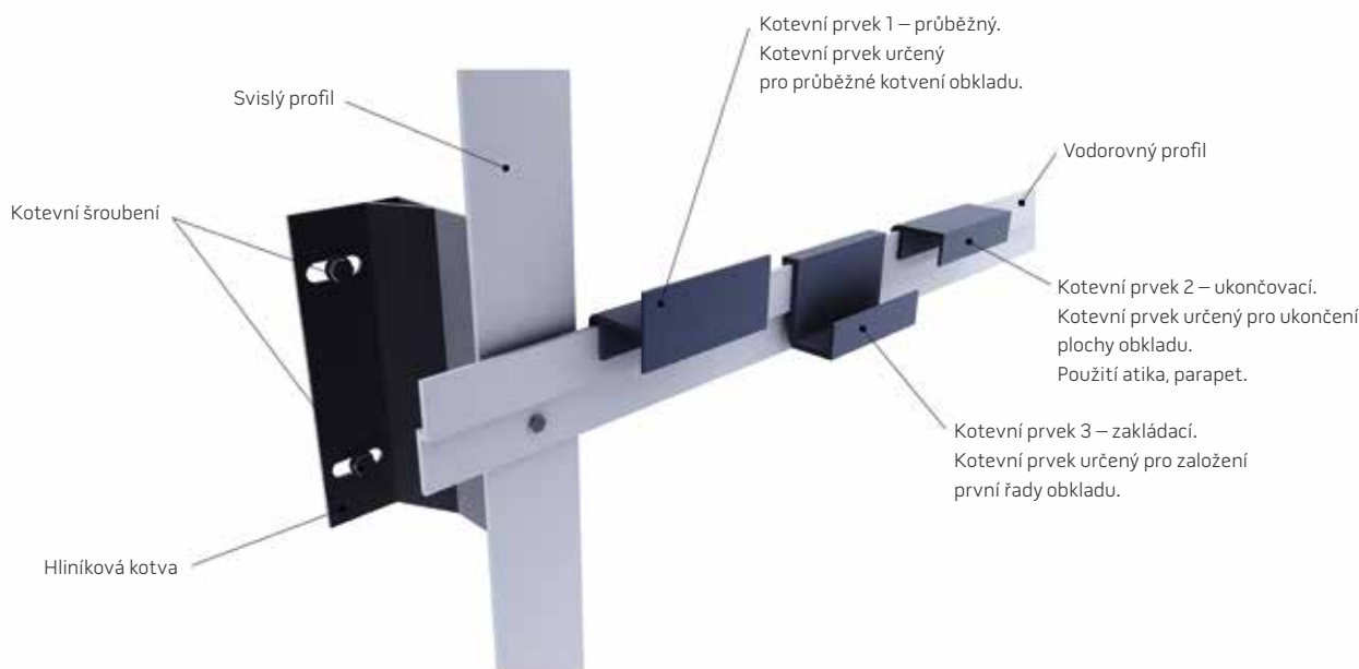
Obr. č. 1 Schéma kotevního systému
