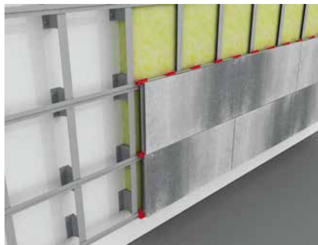
Obr. č. 10 Osazování fasádních desek s vloženou tepelnou izolací a difuzní fólií
